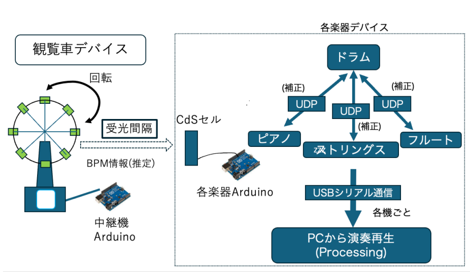
図 20 楽器デバイスのシステム構成図
