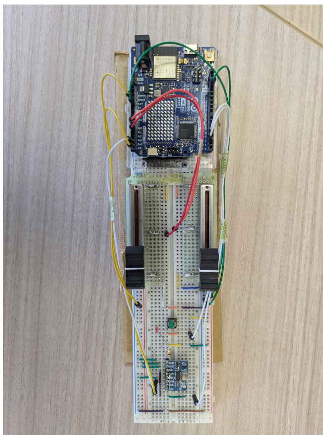
図 25 指揮デバイスの内部実装
