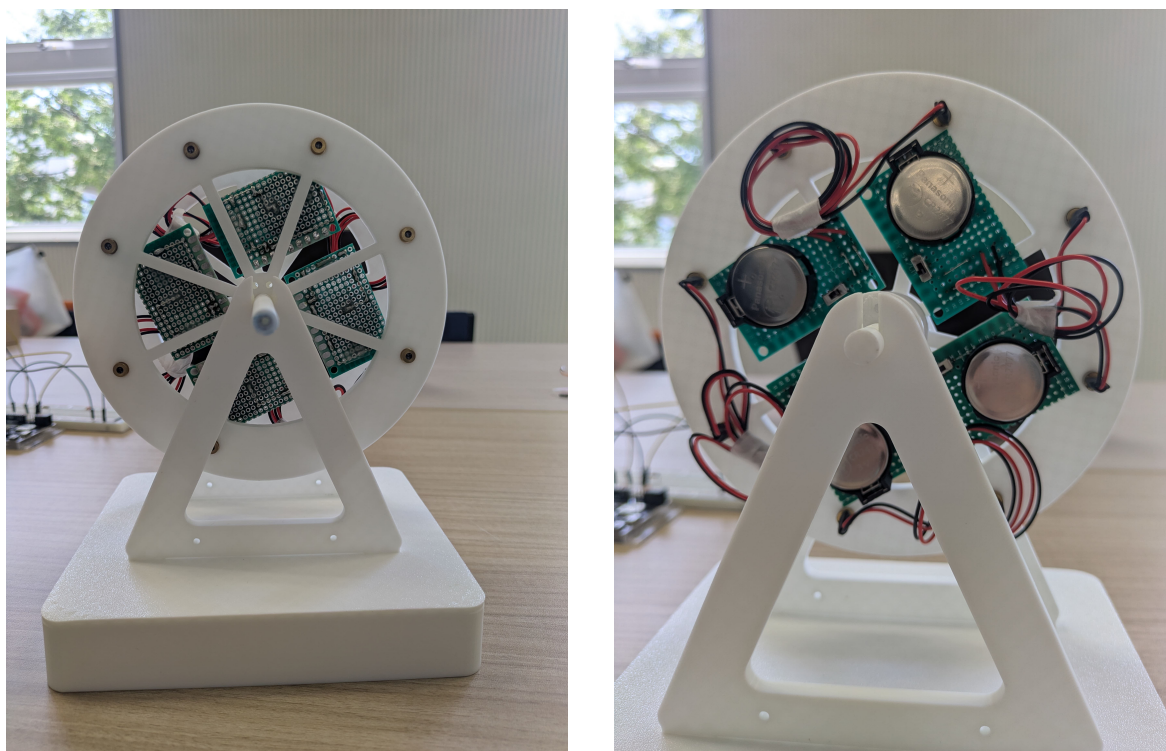
図 30 回転リングへの電池基板の実装（左：正面，右：背面．4 枚の電池基板を中心軸を囲うように十字状の対称配置とし，ボタン電池 CR2477・ホルダー・スライドスイッチを搭載している）
